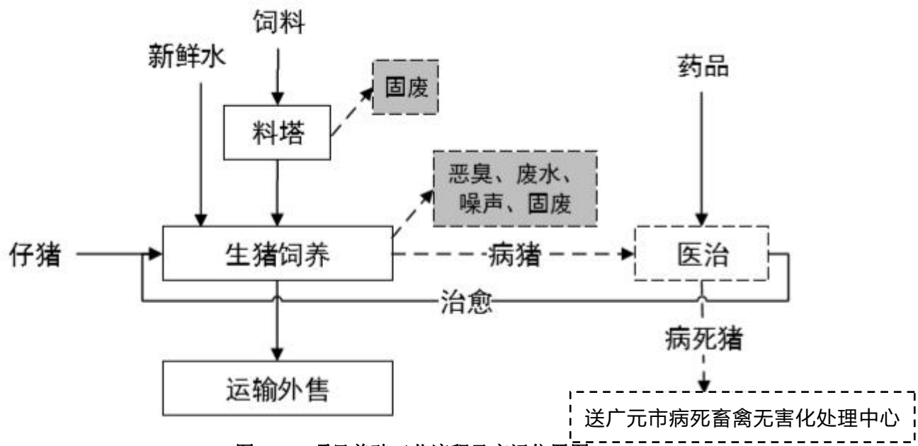
图 3-2 项目养殖工艺流程及产污位置图 本项目产污位置及处置措施见下图所示
