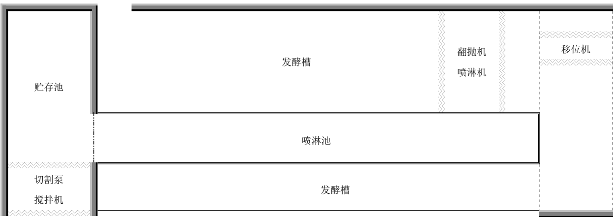
图 6-1 异位发酵床建设示意图
