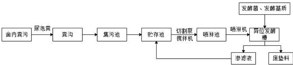
图 5-1 废水处理工艺流程图
