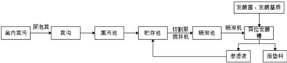
图 3-5 生产废水和粪便处理工艺流程图
