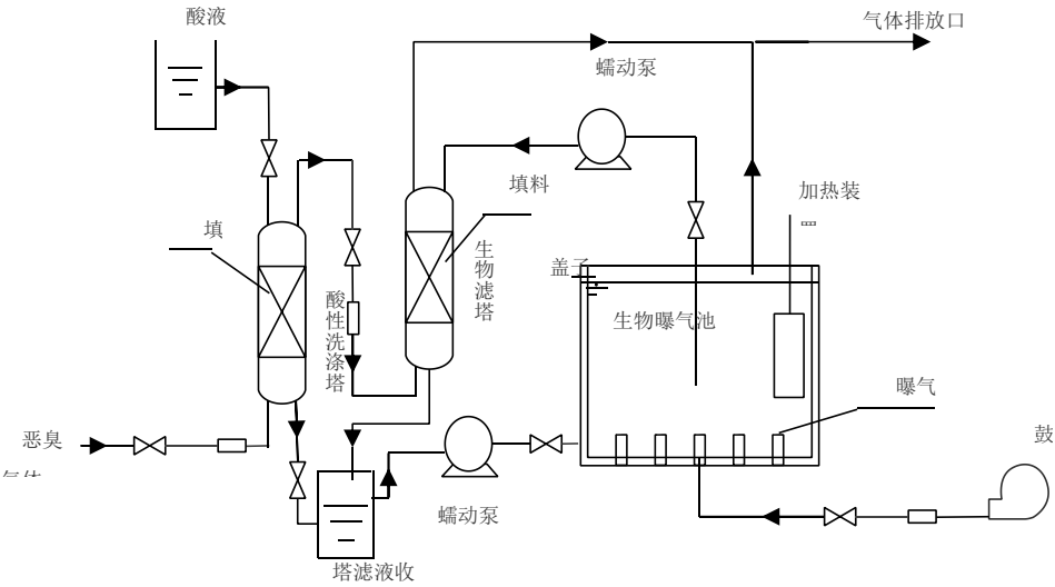
图 6-4 恶臭气体处理工艺流程图
