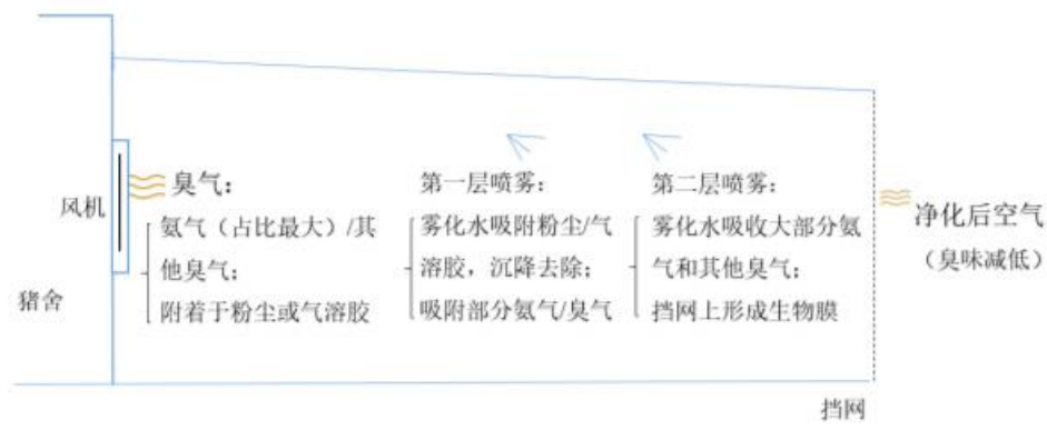
图 6-3 猪舍除臭装置示意图
