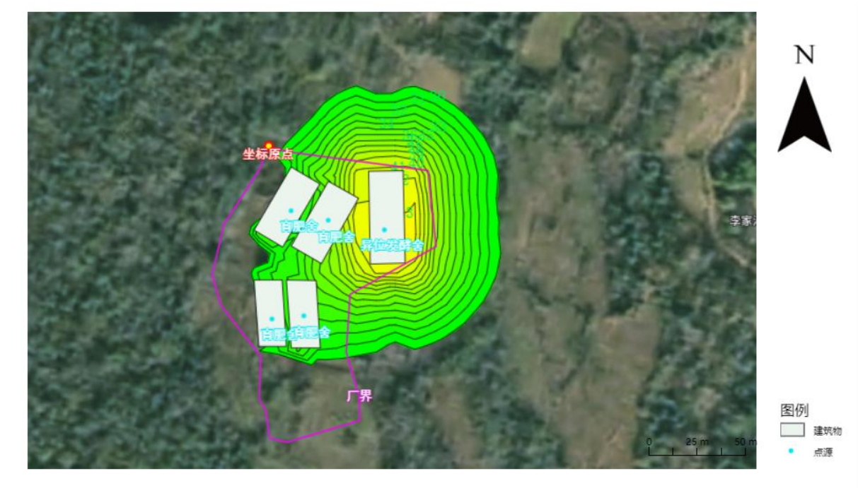
图 5-2 昼间等级声线图
