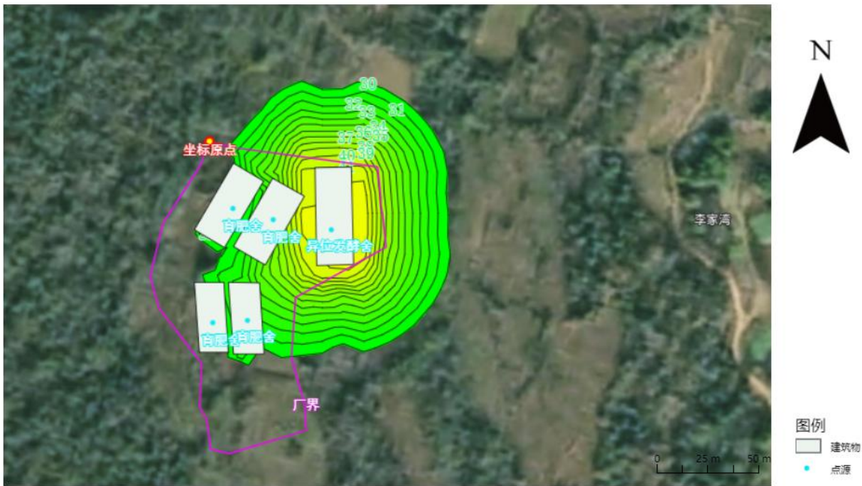
图 5-3 夜间等级声线图
